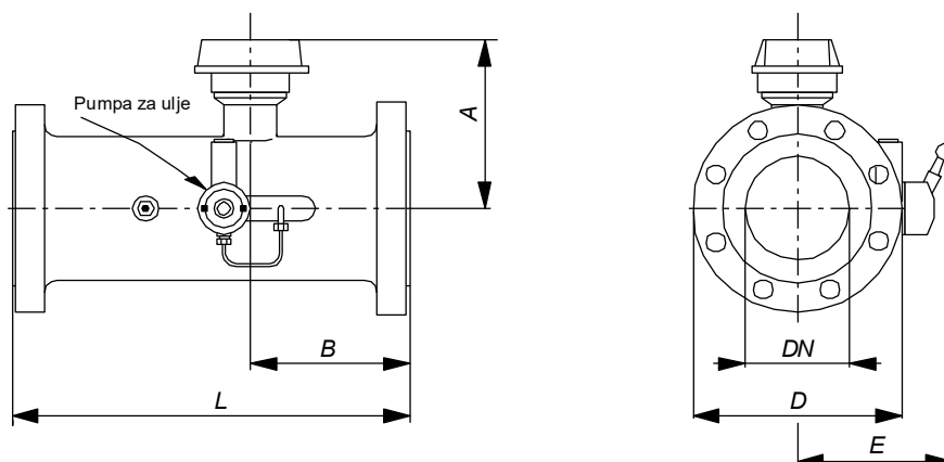
Slika 7. Dimenzije turbinskih plinomjera G-65 do G-4000
