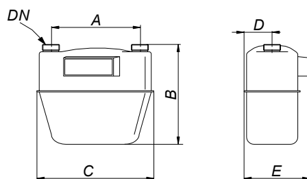
Slika 3. Dimenzije plinomjera G-4, G-6, G-10, G-16 i G-25
