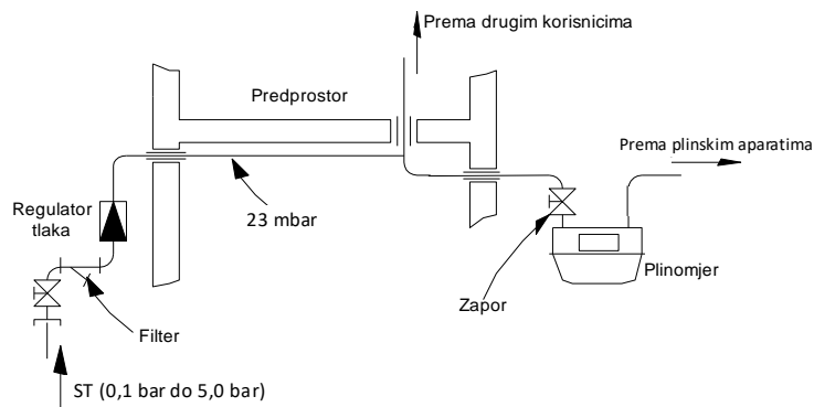
Slika 4. Shematski prikaz plinske instalacije za Q \leq 25 \text{ m}^3/\text{h}
