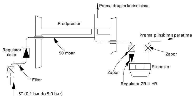
Slika 5. Shematski prikaz plinske instalacije za Q > 25 \text{ m}^3/\text{h}
