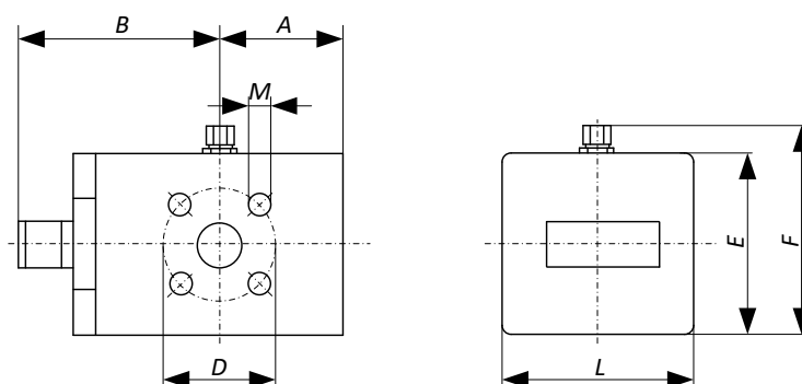
Slika 6. Dimenzije rotacijskih plinomjera G-16 do G-100
