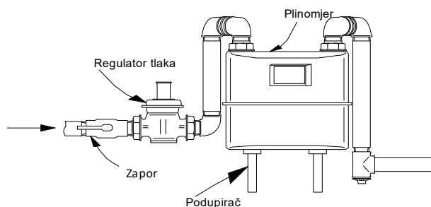
Slika 2. Način ugradnje membranskih plinomjera G-16 i G-25 iznad poda
